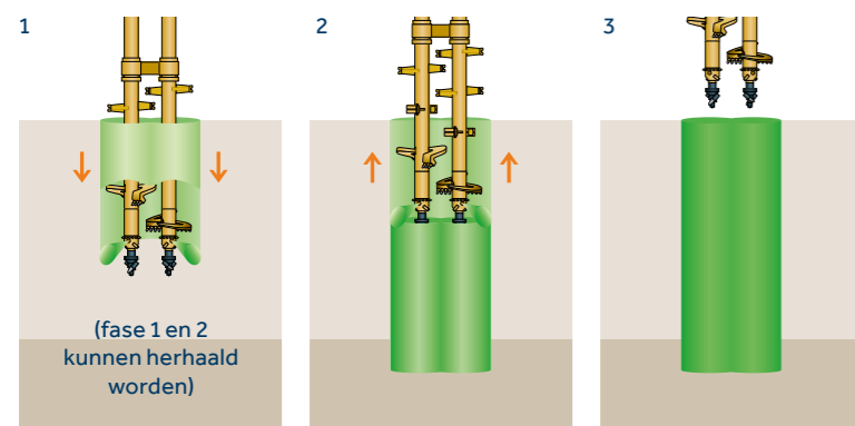
Het nat-mengsysteem
