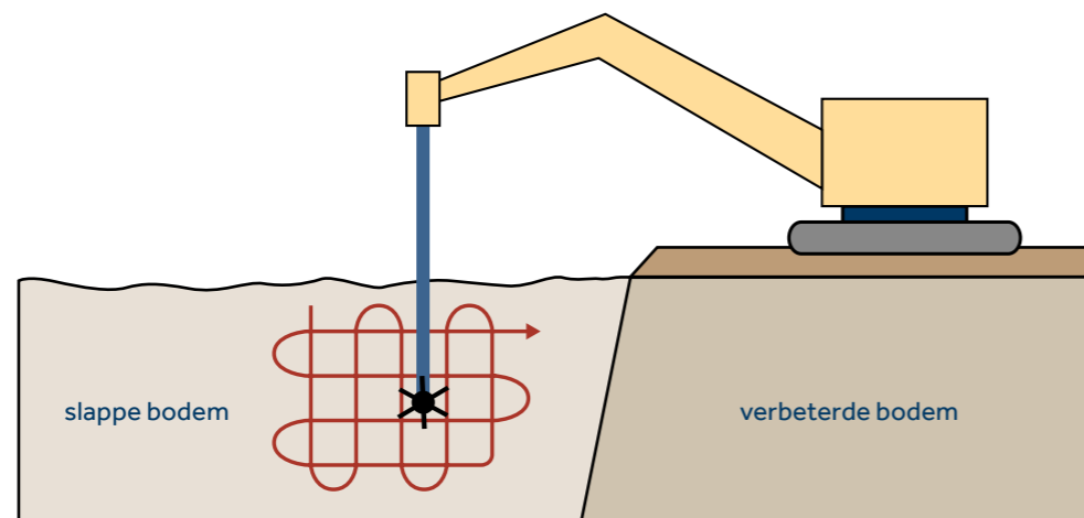
Massastabilisatie procedé
